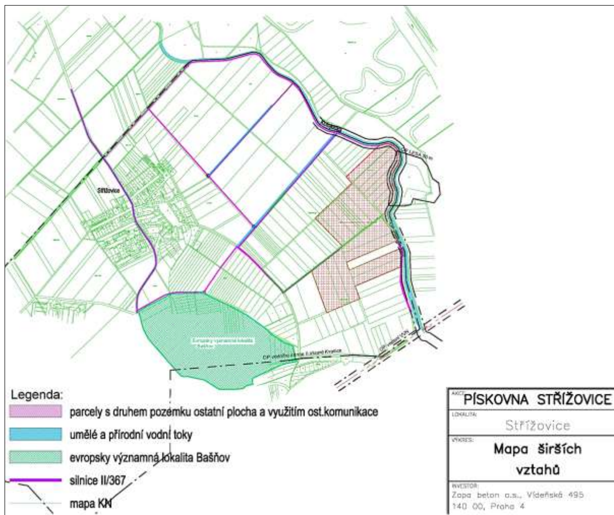
Obr. 29: Schematické situační mapky umístění plánovaného nevýhradního ložiska Střížovice k využití a dopravní napojení do těžebny (severní a jižní trasa s obchvatem obce Střížovice). Nutné je zachování vodního režimu v blízké EVL CZ0723426 Střížovice (bývalá EVL Bašňov)
