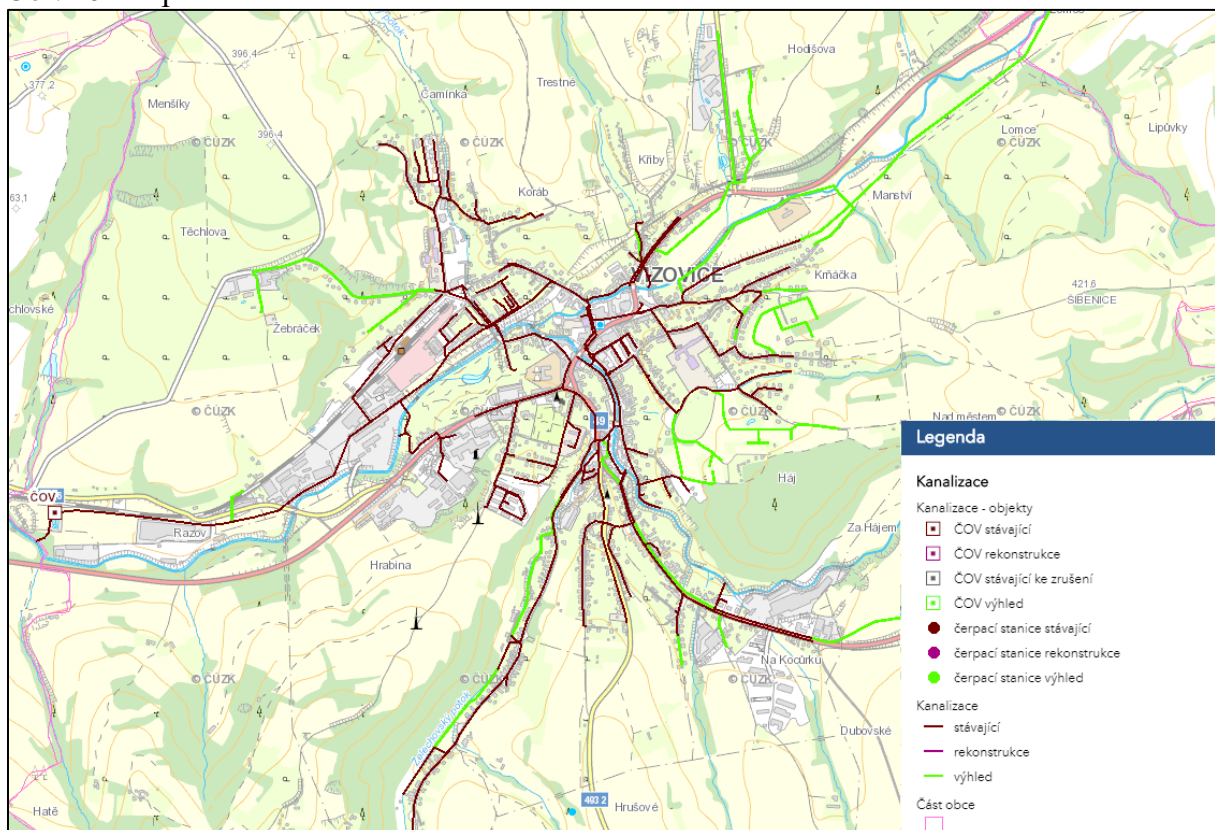
Obr. 10: Mapa kanalizace ve městě Vizovice
