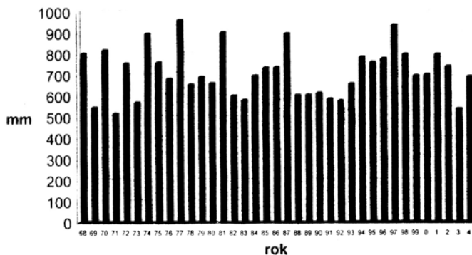
Srážkový úhrn 1968-2004
