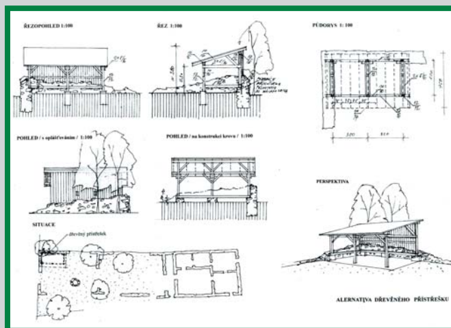
Návrhy přístřešku.
